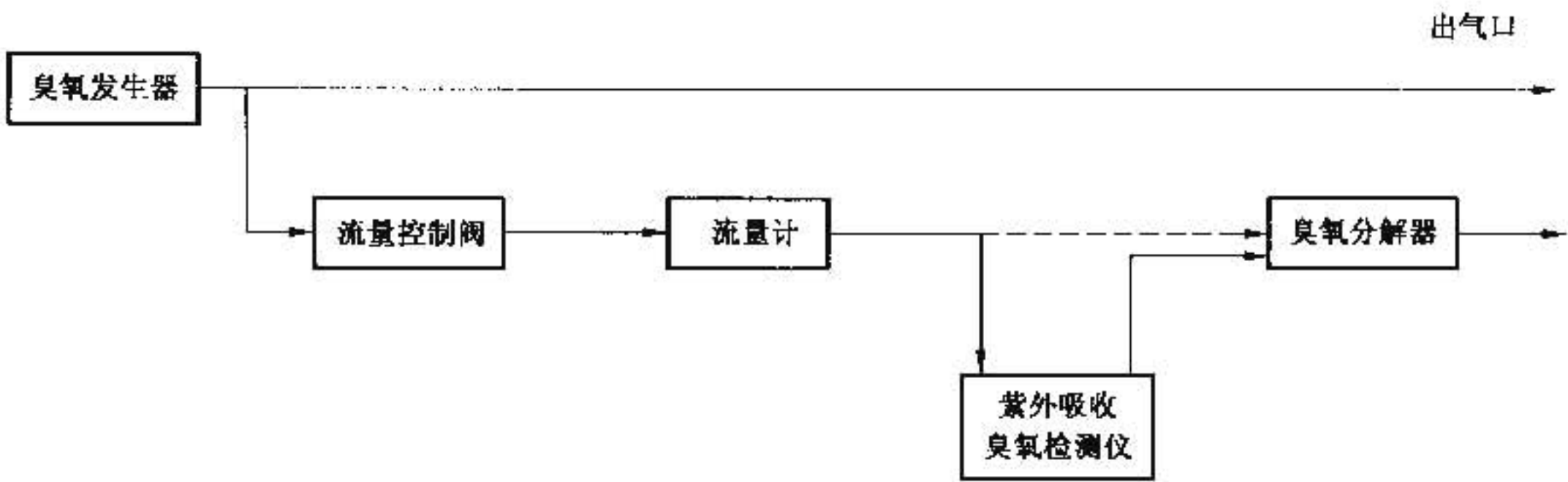
图 A.2 臭氧浓度检测系统示意图
